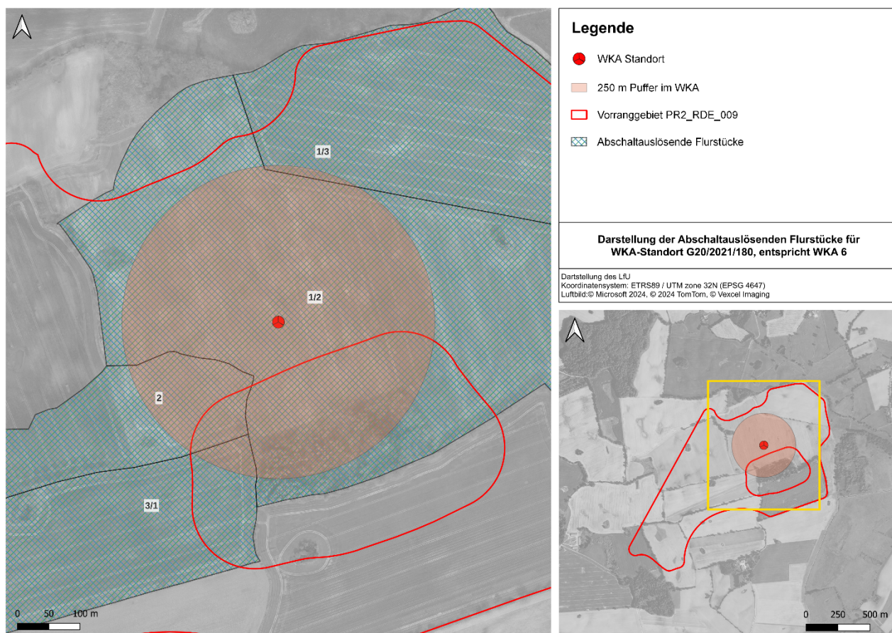
Abbildung 1: Darstellung der abschaltauslösenden Flurstücke für WKA 6 (G20/2021/180)
